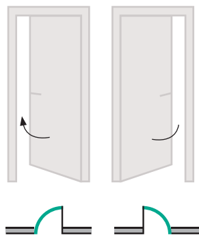
FORDÍTOTT FALCOS AJTÓK BALOS AJTÓ JOBBOS AJTÓ
