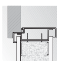
NAGY saroktok beépítése gipszkarton falba
