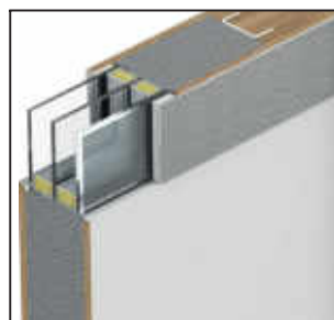
Háromrétegű meleg peremes üvegezéssel – P4 betörésvédelmi osztály, rozsdamentes acél kerettel
