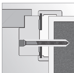
Beépítés purhabbal és dübellel kőműves falba
