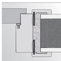
Beépítés a purhabbal kőműves falba
